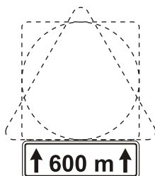
IV-2 Dolžina ceste, na kateri velja pomen znaka
